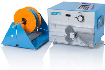
UNIROLL mit UNICUT 8 UNIROLL with UNICUT 8
